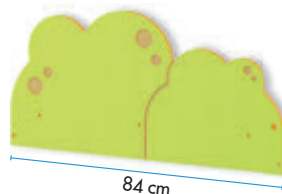
NS8107 Tree
